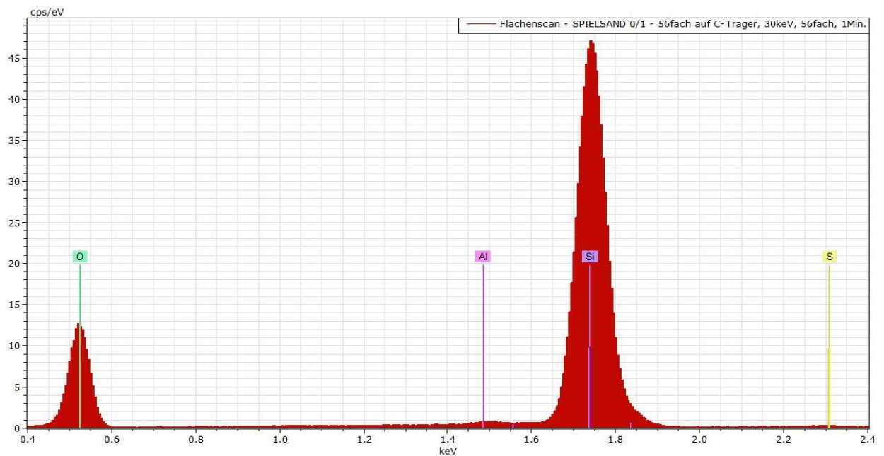
Bild 4: EDX-Flächenscan aus Bild 3
